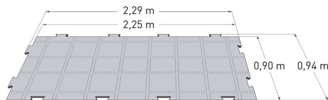
Afmetingen ProPlay®-Sport plaat
