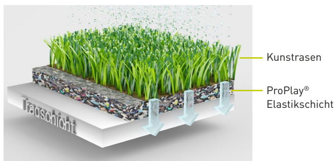
Kunstrasensystem mit ProPlay®-Sport Elastikschiicht
