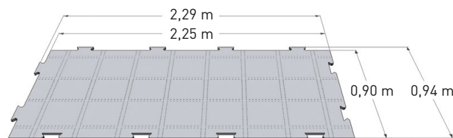
Abmessungen ProPlay®-Sport Platte
