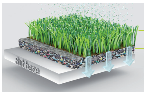
Système de gazon artificiel ProPlay ® -Sport avec absorption des chocs
